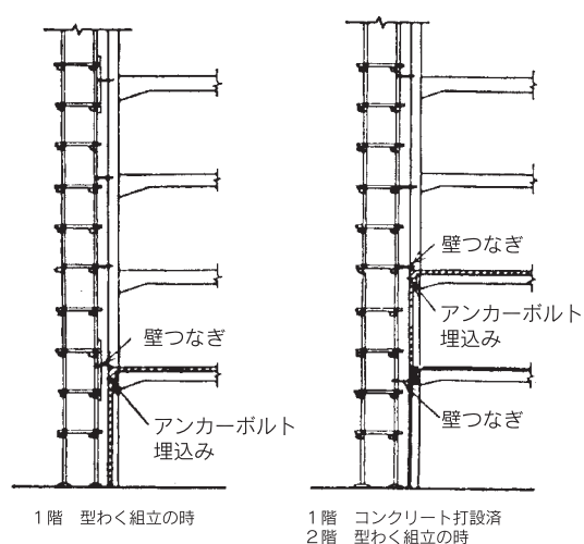
鉄骨鉄筋コンクリート造の場合の壁つなぎ 取付け、盛替え順序
