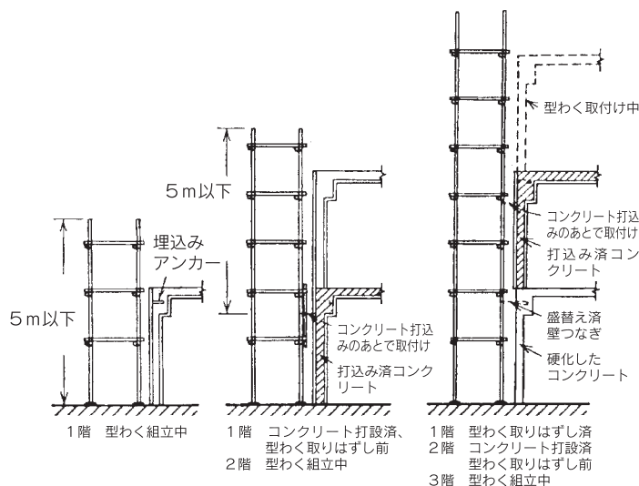
鉄筋コンクリート造の場合の壁つなぎ取付け順序
