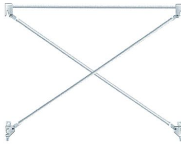
BX-15 φ34×1,500 6.2kg
